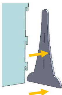
FIG. 2 Inserimento ganci pannello nel piede
